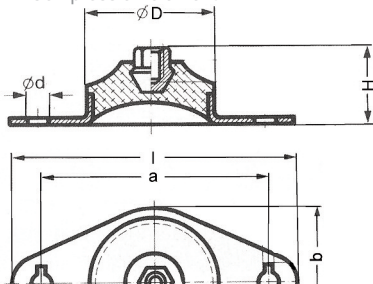
Abb.1 Puffer mit ein oder beidseitigen Aussengewinde. Anti vibration mount with single or double outer thread
