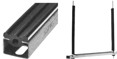
Montagebeispiel mounting example
